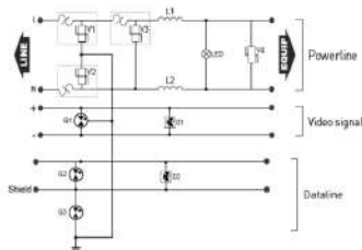
G: газовая трубка D: ограничивающая диодная сеть V: Варистор LED: индикатор состояния L: индуктор
