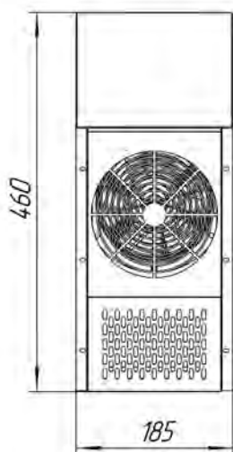
Горячая сторона вентилятора (внешняя)
