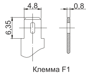
Клемма F1
