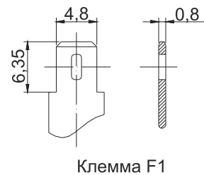
Клемма F1
