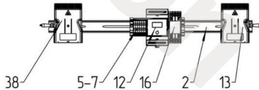
Расположение оборудования на DIN-рейке М 13
