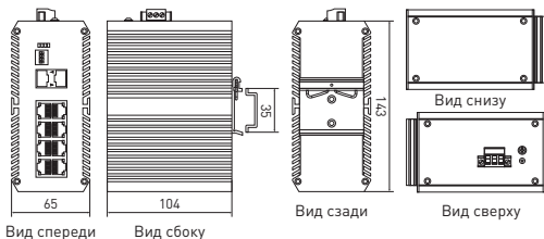
Рис. 1 — Габаритные размеры TSX-U-2GX/SFP-8GTP
